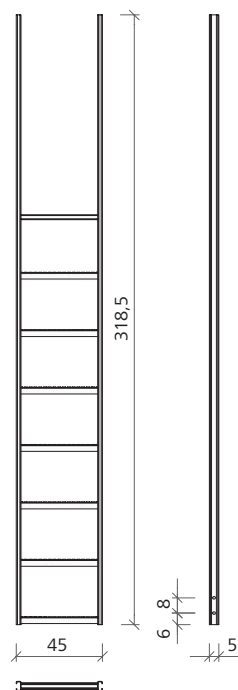
Alaplétra 318
