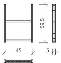
Létrahosszabbító 60
