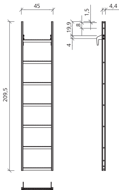
Létrahosszabbító 210
