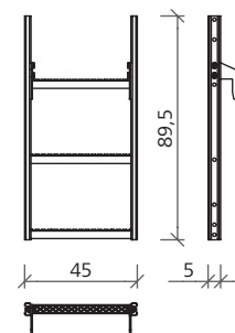
Létrahosszabbító 90
