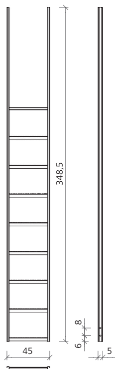
Alaplétra 348
