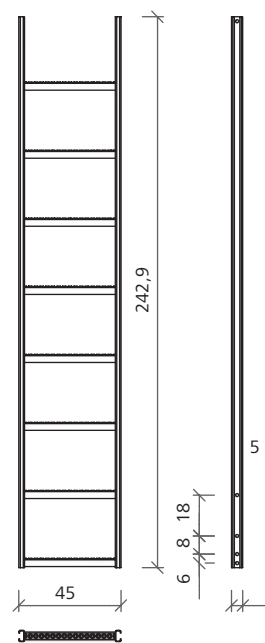
Alaplétra 243
