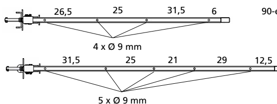
125-ös betonozó konzol
