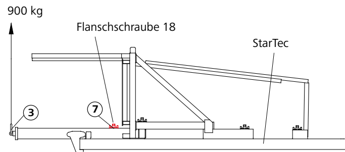
Abb. 6 ST-Hubarm 900 SB
