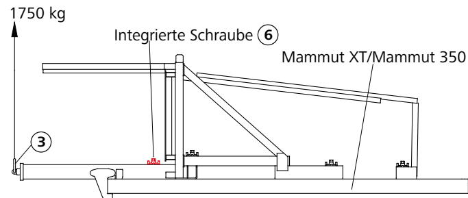
Abb. 5 M-Hubarm 1750 SB
